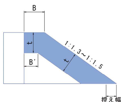
傾斜堤被覆形式
